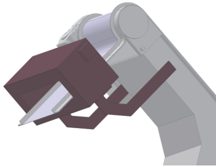
p.m. Rutschförderer mit Entmagnetisierspule
